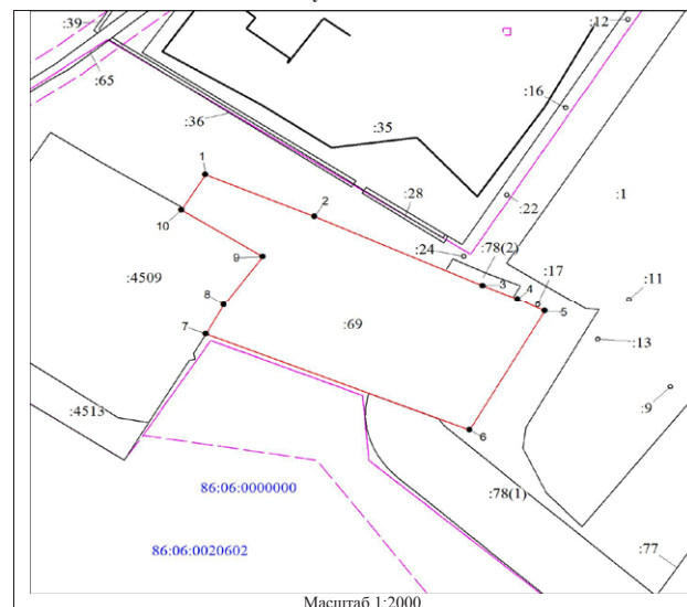
Схема расположения границ публичного сервитута участок №1
